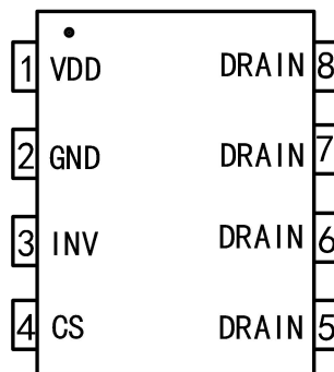
SOP8 Package
